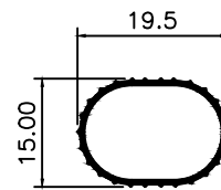
MV-024 0,100 Kg/m
