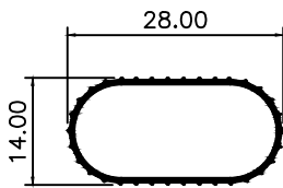
MV-023 0,125 Kg/m
