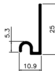
DS-240 0,145 Kg/m
