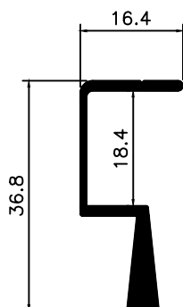
MV-038 0,320 Kg/m
