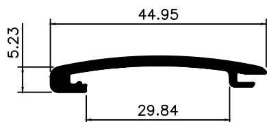
DS-025 0,310 Kg/m
