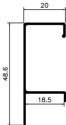
MV-080 0,240 Kg/m
