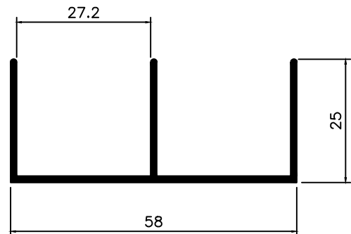
MV-011 0,432 Kg/m
