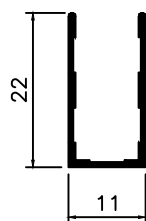
BX-102 0,122 Kg/m
