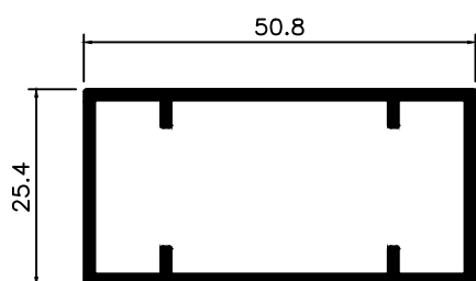
DS-063 0,630 Kg/m
