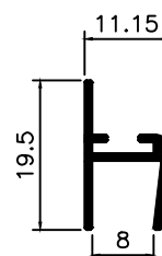
BX-122 0,130 Kg/m
