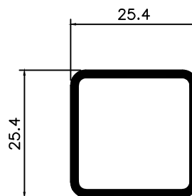
TQ-006CR 0,400 Kg/m
