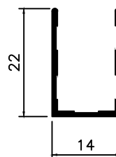
BX-103 0,140 Kg/m
