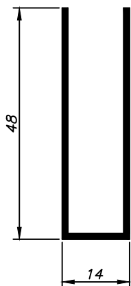
PU-048 0,365 Kg/m
