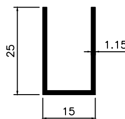
PU-004 0,210 Kg/m
