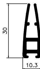
PE-008 0,320 Kg/m
