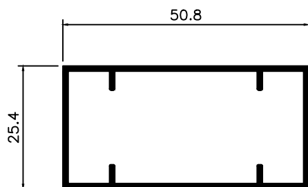
RF-043 0,450 Kg/m
