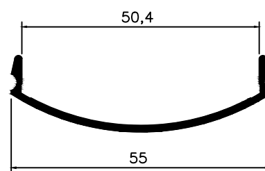
GR-074 0,250 Kg/m
