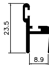
BX-186 0,200 Kg/m
