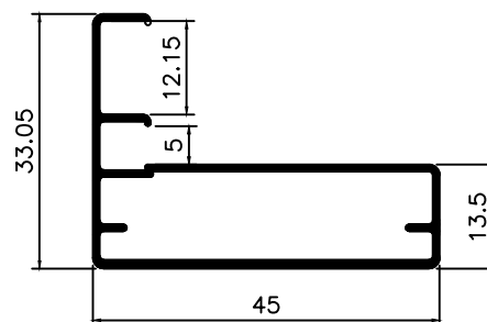
MV-037 0,420 Kg/m
