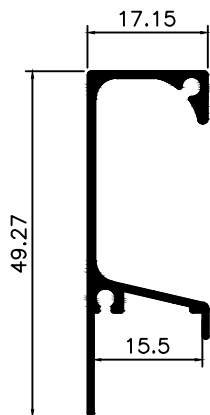
MV-045 0,320 Kg/m
