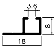
TS-014 0,087 Kg/m
