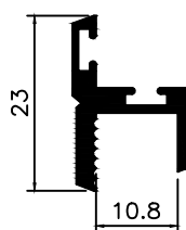
BX-192 0,240 Kg/m
