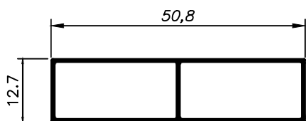
BT-006 0,260 Kg/m
