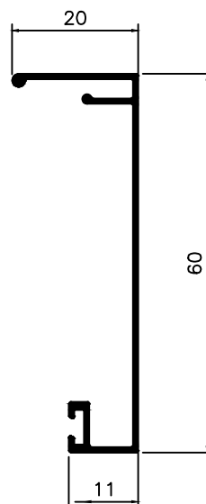
BX-135 0,275 Kg/m
