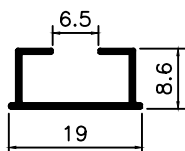
TS-001 0,100 Kg/m
