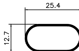
DS-056 0,136 Kg/m
