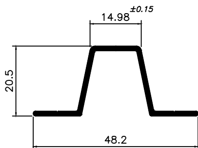
DS-121 0,510 Kg/m
