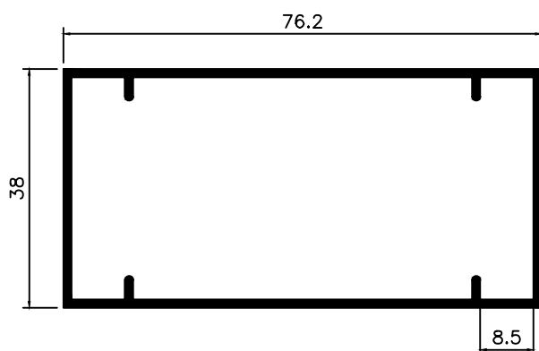
DS-052 0,837 Kg/m
