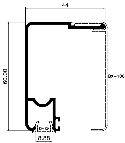
BX-105 0,535 Kg/m
