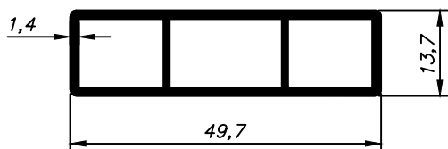
MV-007 0,528 Kg/m
