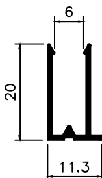
DS-474 0,150 Kg/m
