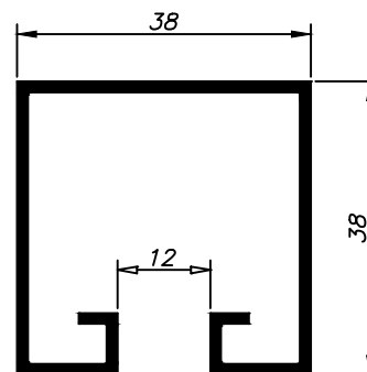
DS-471 0,595 Kg/m
