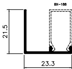
BX-187 0,145 Kg/m
