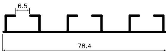
TS-003 0,330 Kg/m
