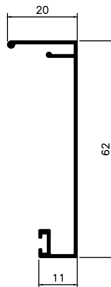
BX-128 0,280 Kg/m
