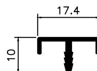
MV-019 0,108 Kg/m
