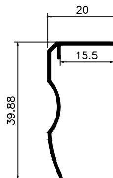
MV-049 0,190 Kg/m
