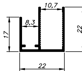
BX-141 0,220 Kg/m
