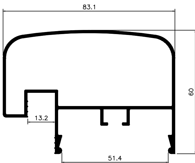
GR-083 1,187 Kg/m
