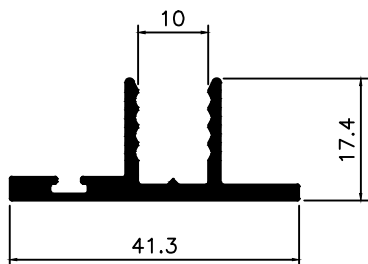
VT-001 0,420 Kg/m
