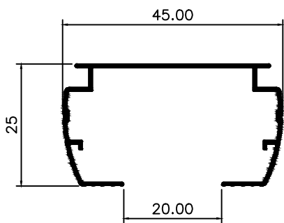
PE-001 0,256 Kg/m
