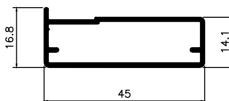
MV-065 0,420 Kg/m
