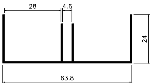
MV-058 0,335 Kg/m
