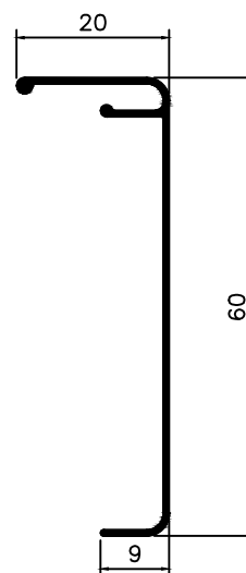
BX-106 0,240 Kg/m
