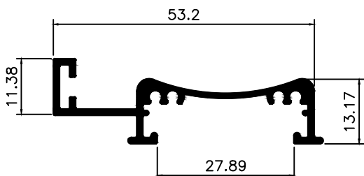
PE-005 0,450 Kg/m
