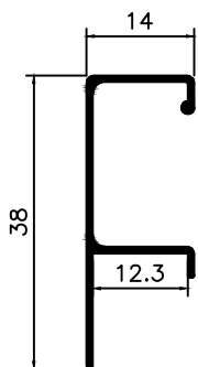
MV-050 0,180 Kg/m
