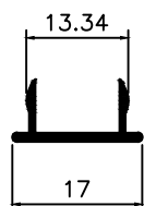
BX-190 0,100 Kg/m
