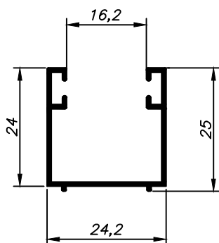
BX-139 0,238 Kg/m
