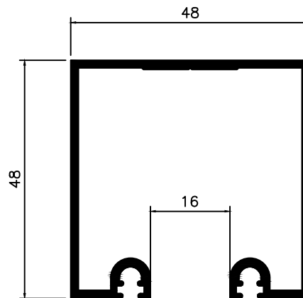
DS-086 0,850 Kg/m
