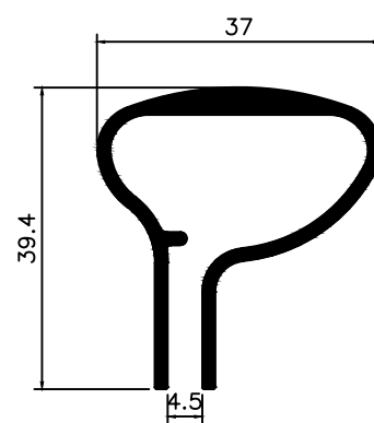
DS-123 0,650 Kg/m
