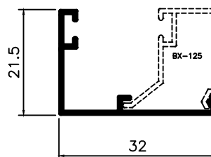
BX-126 0,198 Kg/m
