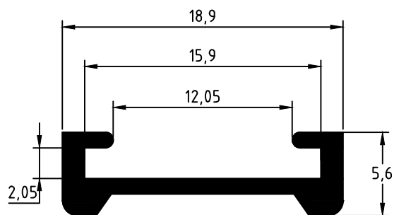
MAX-003 0,130 Kg/m
