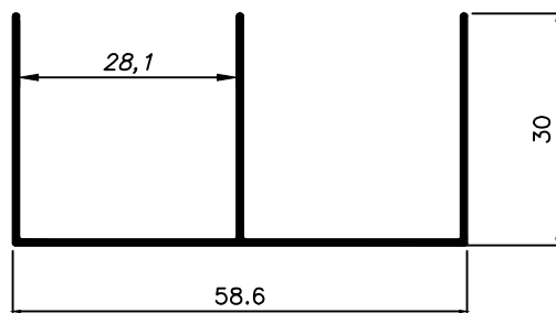
MV-057 0,325 Kg/m
