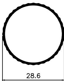
TR-200 0,207 Kg/m
