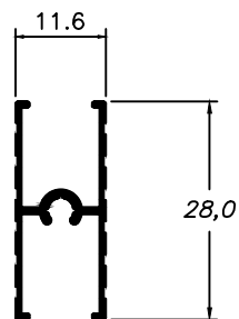
BX-053 0,172 Kg/m
