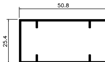
DS-051 0,520 Kg/m
