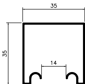
DS-230 0,340 Kg/m
