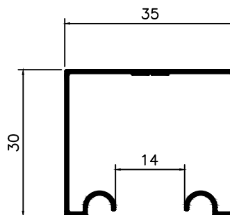
DS-229 0,290 Kg/m
