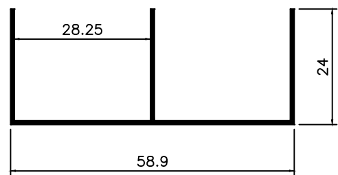
MV-034 0,290 Kg/m
