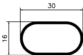
DS-054 0,213 Kg/m
