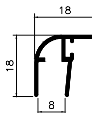
BX-138 0,150 Kg/m
