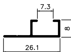
TS-015 0,110 Kg/m
