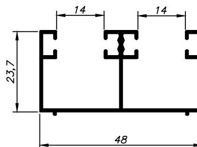
BX-140 0,430 Kg/m
