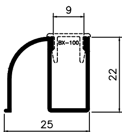
BX-110 0,230 Kg/m
