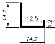
MV-046 0,080 Kg/m
