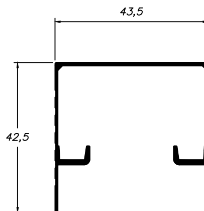
BX-183 0,396 Kg/m
