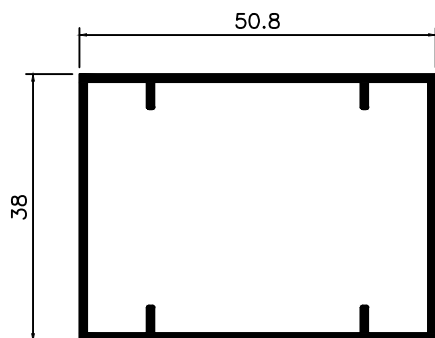
DS-050 0,561 Kg/m
