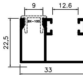
BX-107 0,330 Kg/m
