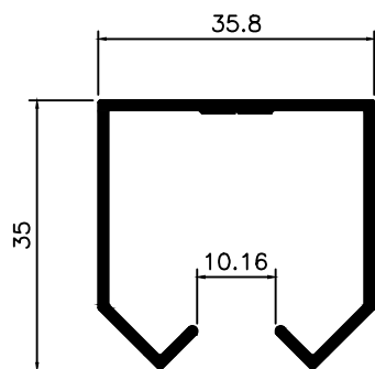
DS-473 0,440 Kg/m
