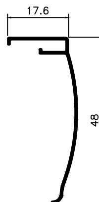
BXE-001 0,180 Kg/m
