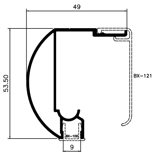
BX-119 0,521 Kg/m
