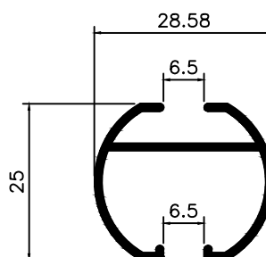
TS-009 0,325 Kg/m
