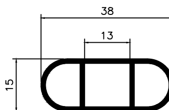
MV-008 0,386 Kg/m
