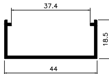
GR-079 0,280 Kg/m
