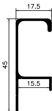
MV-022 0,260 Kg/m
