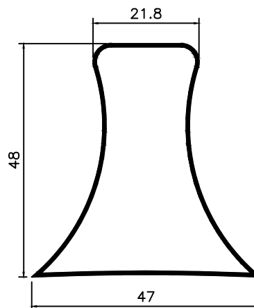
RP-001 0,340 Kg/m
