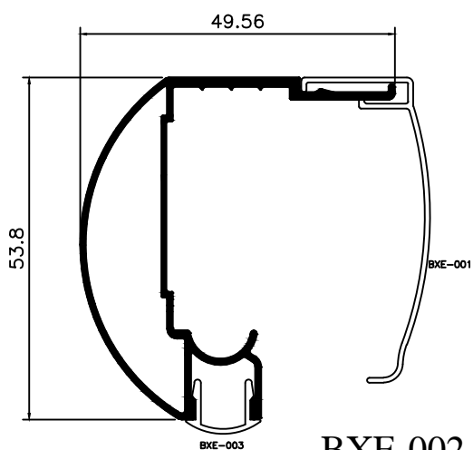
BXE-002 0,550 Kg/m
