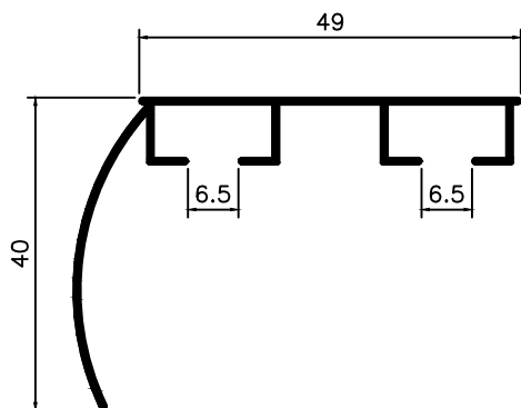
TS-005 0,345 Kg/m
