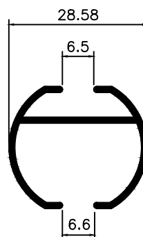
TS-011 0,320 Kg/m
