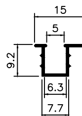
MV-021 0,065 Kg/m
