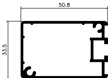
GR-077 0,745 Kg/m
