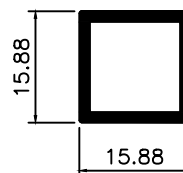
TQ-018 0,236 Kg/m
