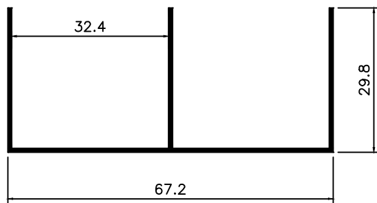
MV-033 0,345 Kg/m
