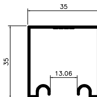
DS-236 DS-237 0,400 Kg/m 0,480 Kg/m
