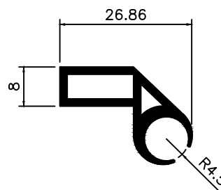
DS-105 0,350 Kg/m
