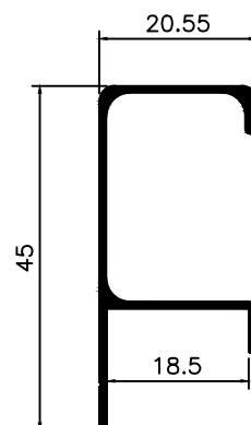
MV-048 0,270 Kg/m
