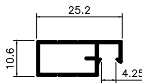
25-273 0,195 Kg/m
