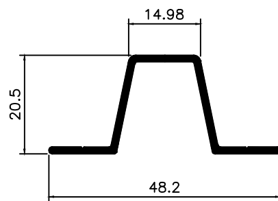
DS-120 0,368 Kg/m
