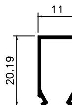
BX-188 0,130 Kg/m
