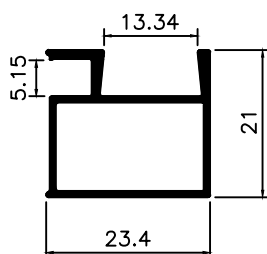
MV-076 0,260 Kg/m
