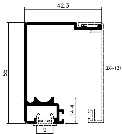
BX-130 0,540 Kg/m
