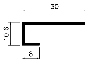
DS-225 0,150 Kg/m
