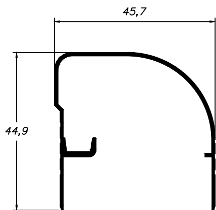
BX-055 0,375 Kg/m
