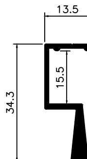
MV-060 0,305 Kg/m
