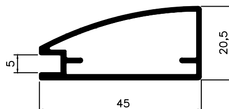
MV-026 0,500 Kg/m
