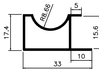
MV-041 0,260 Kg/m
