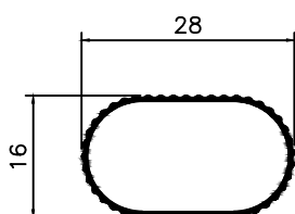
MV-055 0,120 Kg/m
