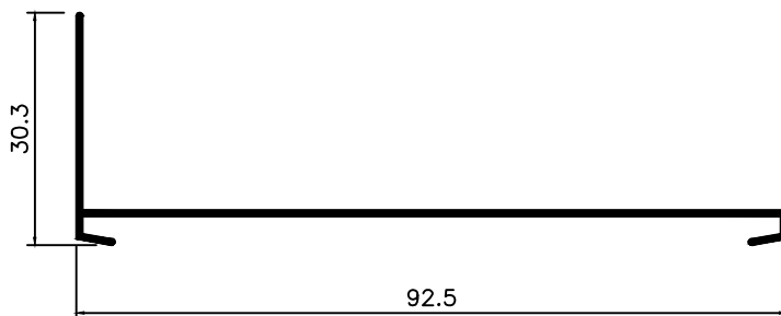
PE-002 0,290 Kg/m
