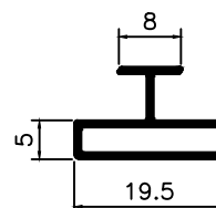
MV-030 0,160 Kg/m
