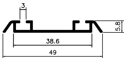
MV-012 0,238 Kg/m
