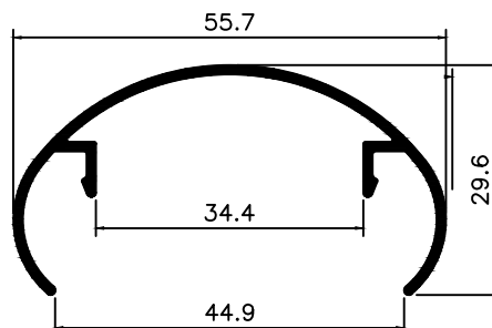
GR-078 0,385 Kg/m
