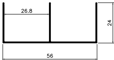
MV-056 0,285 Kg/m
