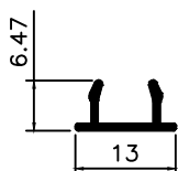
BX-124 0,060 Kg/m
