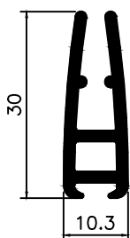
PE-004 0,370 Kg/m
