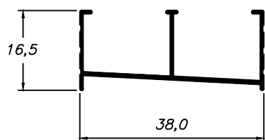
BX-052 0,185 Kg/m
